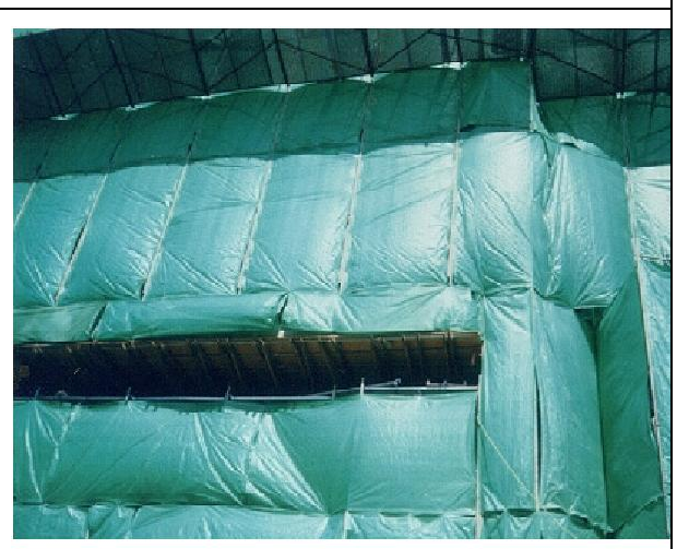
(D) SRC 結構體設置防塵布
